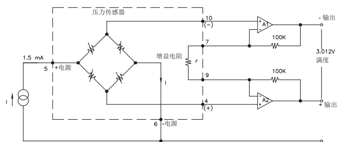
应用原理图
