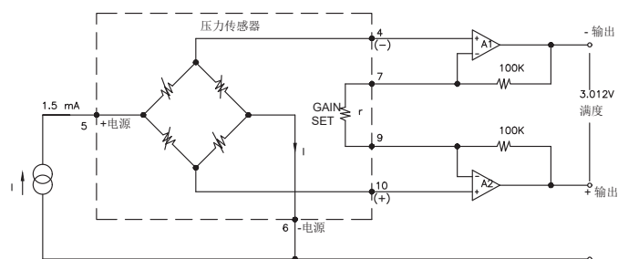
应用原理图
