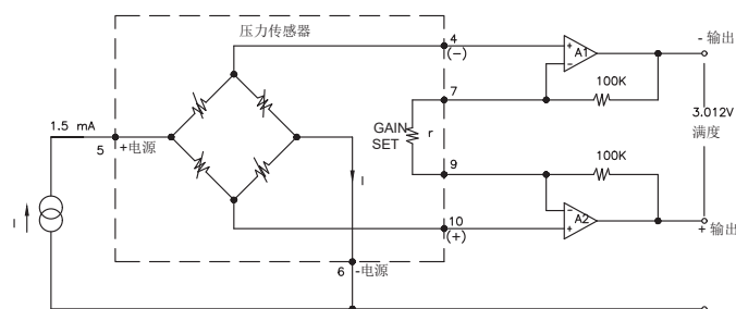
应用原理图
