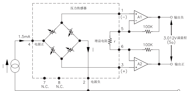
应用电路
