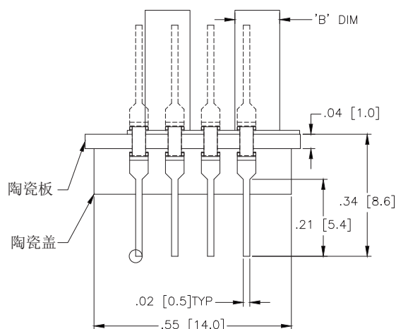
金属管和陶瓷管封装尺寸，陶瓷板电路展示为LP1230
