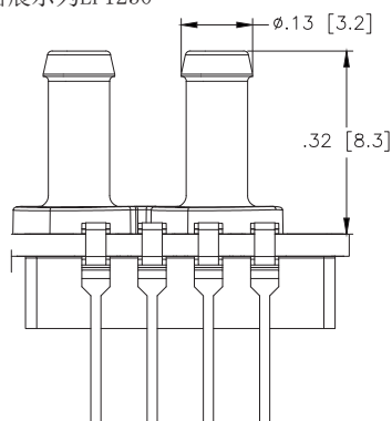
塑胶管封装尺寸，陶瓷板电路展示为LP1230
